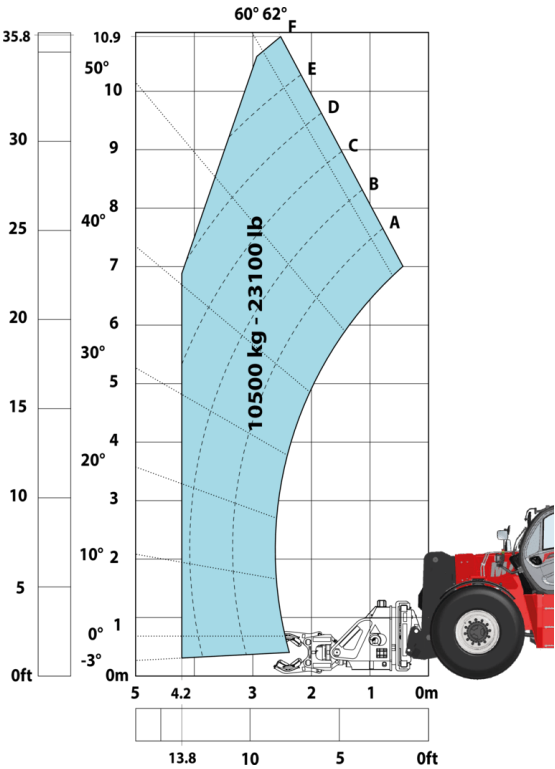
Machine sur pneus avec pince à verins CH 10 (Metric)
