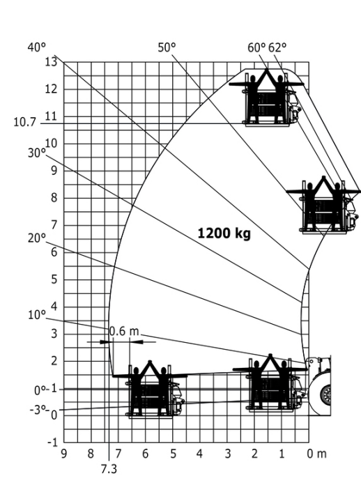
Machine sur pneus avec panier mine (Métric)
